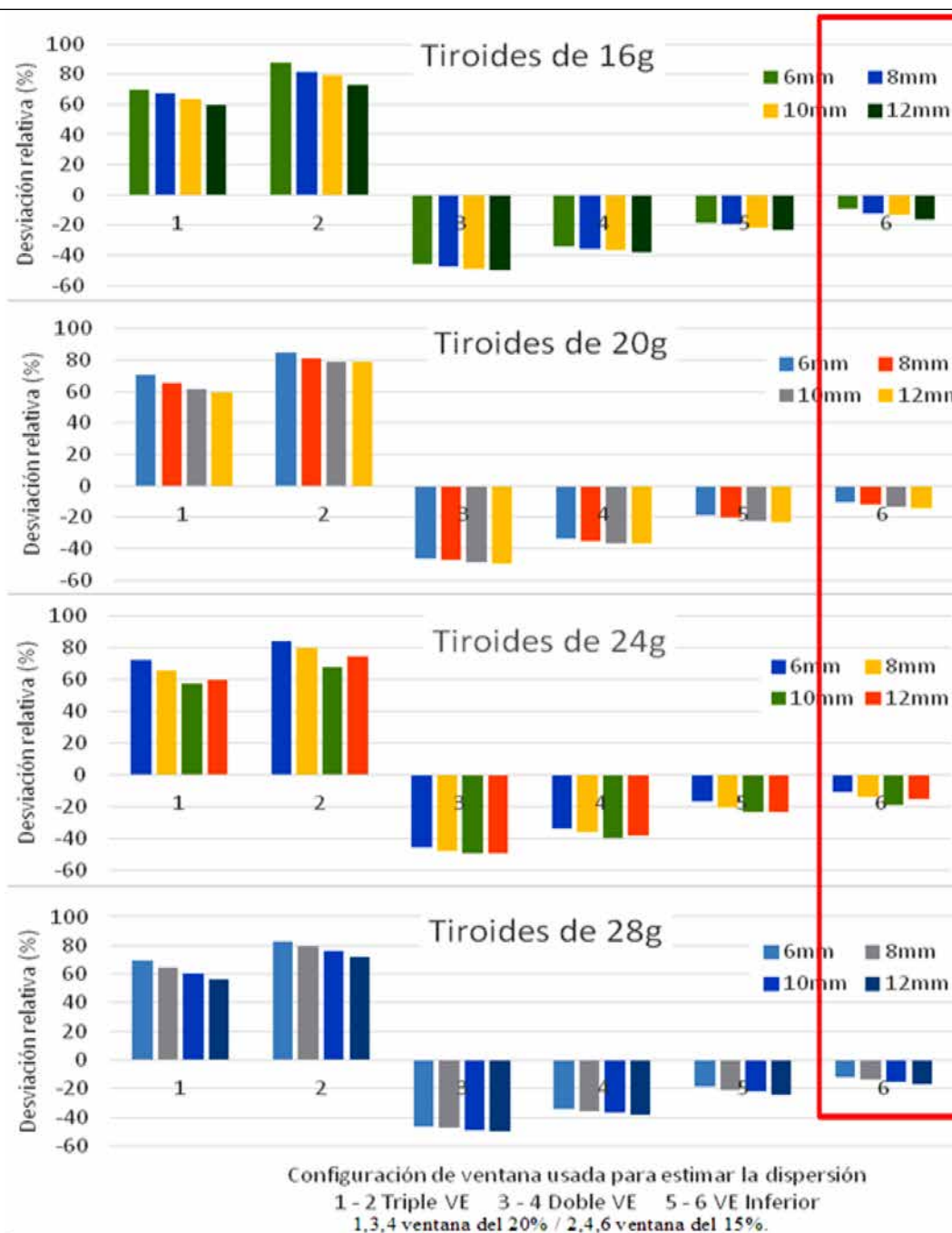
Figura 1. Resultados del estudio de evaluación por Monte Carlo de los métodos de corrección de dispersión con ^{131}\text{I} empleando colimador pinhole en estudios de tiroides [24].
