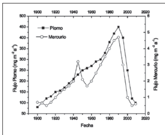
Figura 4. Evolución histórica de los flujos de mercurio y plomo a los sedimentos de la bahía de la Habana
