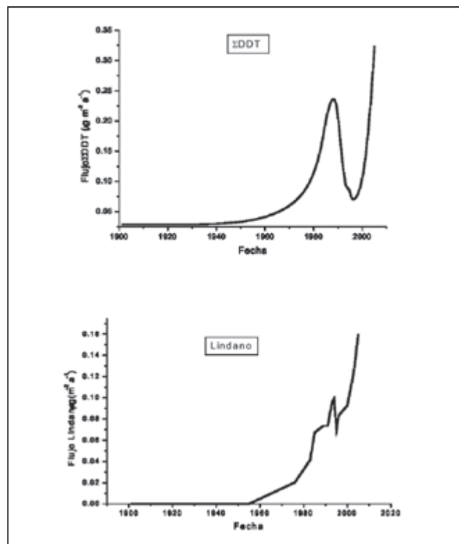
Figura 5. Flujos de DDT y lindano a los sedimentos del estuario del río La Coloma, en el Golfo de Batabanó.
