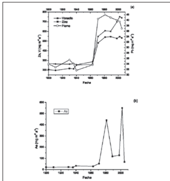
Figura 2. Flujo de plomo, zinc, vanadio y arsénico a los sedimentos en la Bahía de Cienfuegos.
