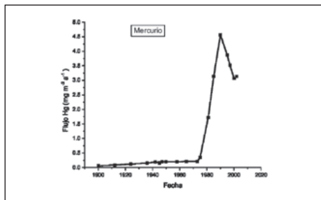
Figura 3. Evolución de la contaminación por mercurio del estuario del río Sagua.
