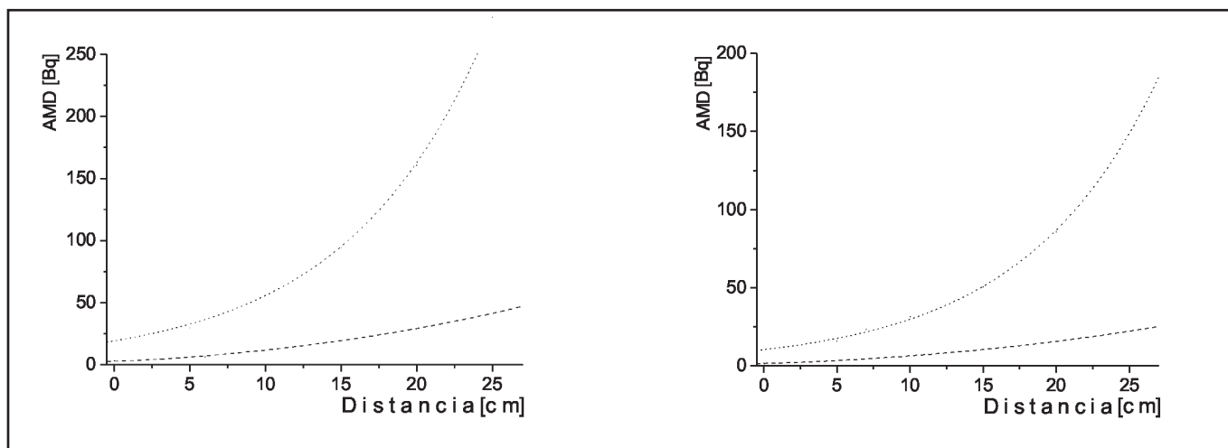
Figura 2a. Comportamiento de la AMD con la distancia. Línea discontinua (Phoswich). Línea punteada (centellante) para el ^{129}\text{I}
