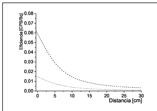
Figura 1. Comportamiento de la \eta con la distancia. Línea discontinua (Phoswich), línea punteada (centellante)
