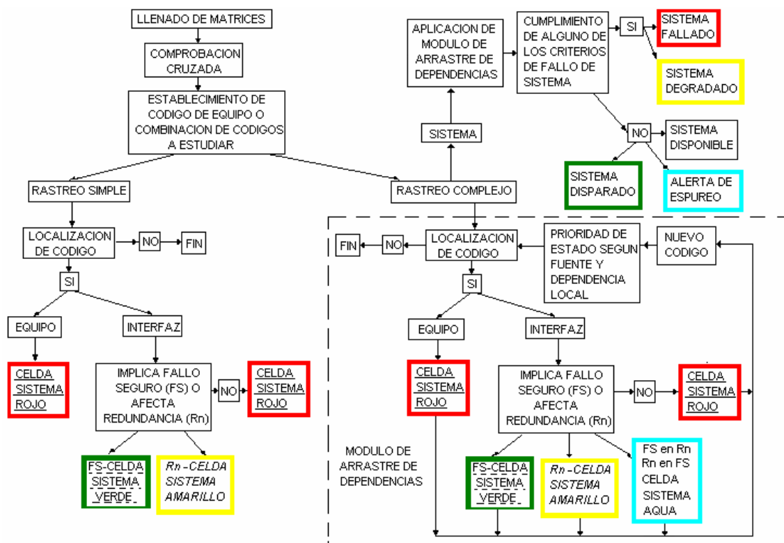
Figura 1. Algoritmo de control de configuraciones peligrosas.
