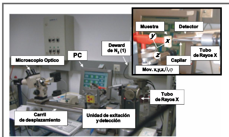
Figura 2. Instalación de sistema de micro-fluorescencia de rayos X ( \mu XRF).
