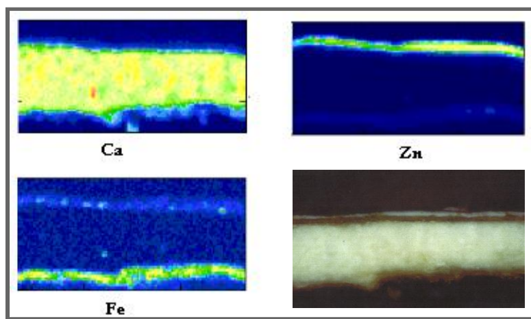
Figura 4. Mapa de distribución de elementos μXRF de la muestra I.4, donde se resuelve el estrato blanco (blanco de zinc) y el estrato carmelita pigmentado con ocre (óxido de hierro) de espesores de 25 \mu\text{m} y 30 \mu\text{m} .
