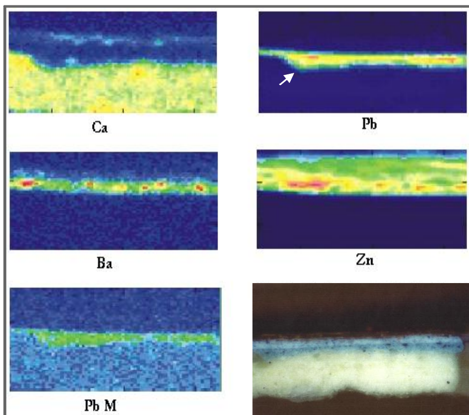
Figura 5. Mapas de distribución elemental por \mu FRX de la muestra I.6.
