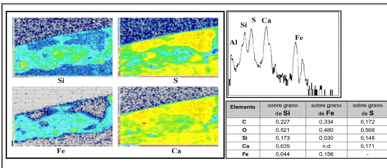
Figura 6. Mapas de distribución elemental y espectro de \mu PIXE de la muestra III.1 y valores de concentraciones (normalizados a 1) determinados por \mu PIXE-RBS.
