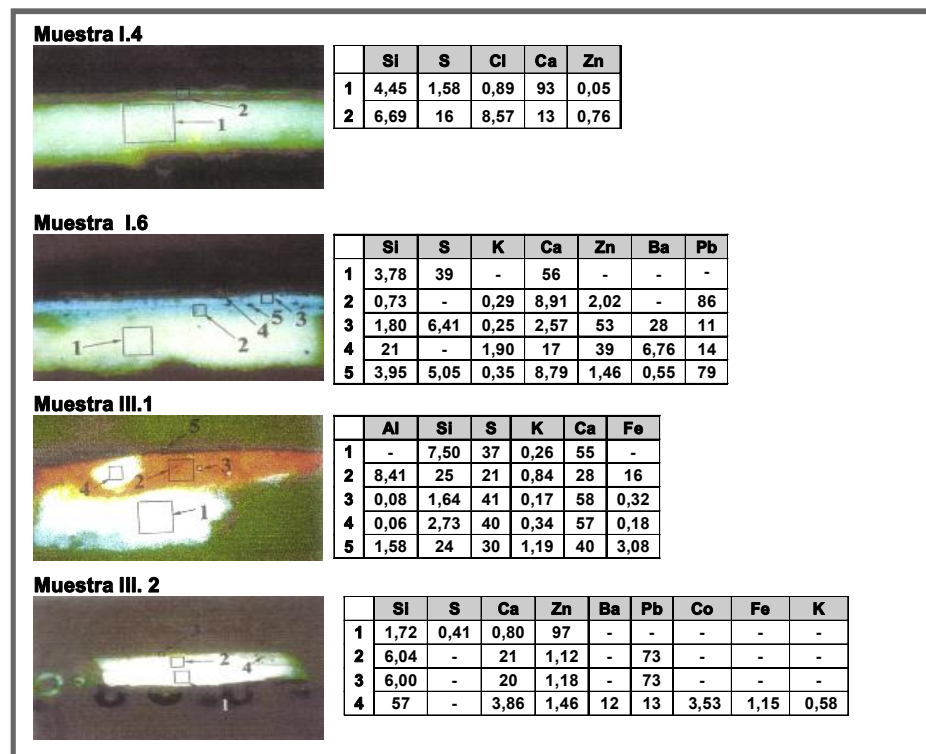
Figura 3. Fotomicrografías de las muestras de secciones transversales de las policromías estudiadas al microscopio óptico con indicación de puntos donde se determinaron los valores de concentración (en %) por SEM-EDX.
