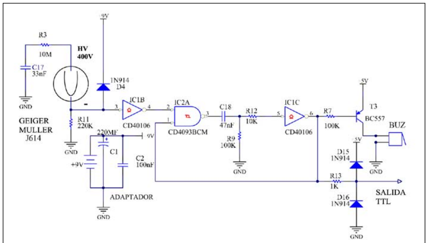
Figura 4. Circuito del Geiger-Muller e interfaz de salida al ATmega88.
