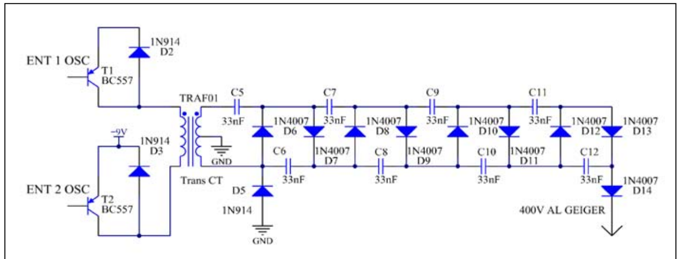
Figura 3. Fuente de Alto Voltaje para el detector Geiger-Müller.
