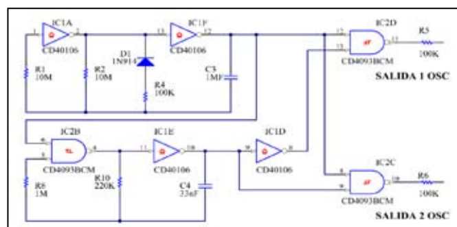
Figura 2. Oscilador de la sección analógica del contador Geiger.
