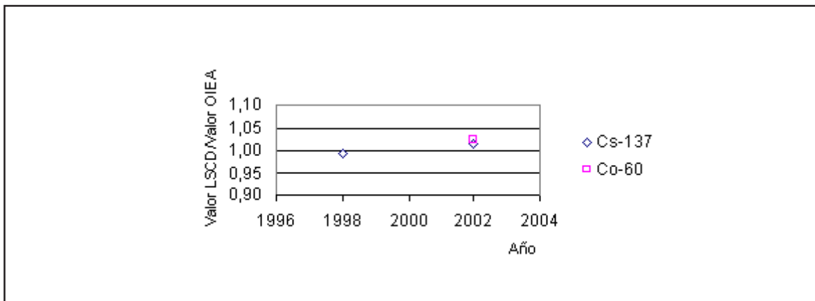
Figura 1. Auditorías postales del OIEA al LSCD de Cuba en haces de 137 Cs y 60 Co para niveles de protección radiológica.
