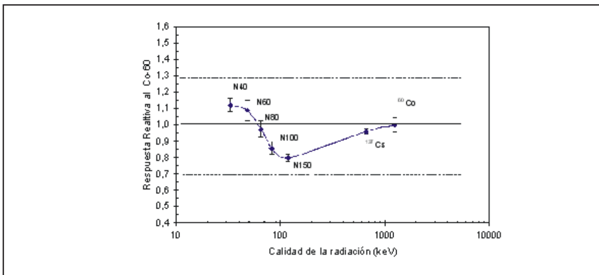
Figura 4. Respuesta de los dosímetros en función de la energía de la radiación fotónica.
