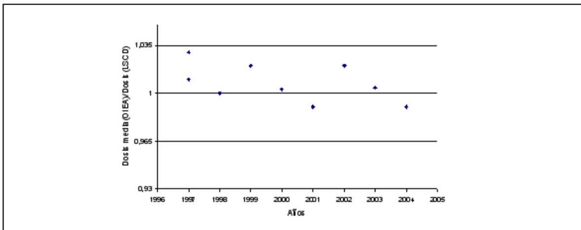
Figura 2. Resultados de las auditorías del OIEA en haces de 60 Co a niveles de radioterapia en el período 1997-2004.
